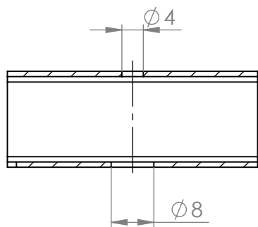
PRZEKRÓJ A-A SKALA 1 : 1
